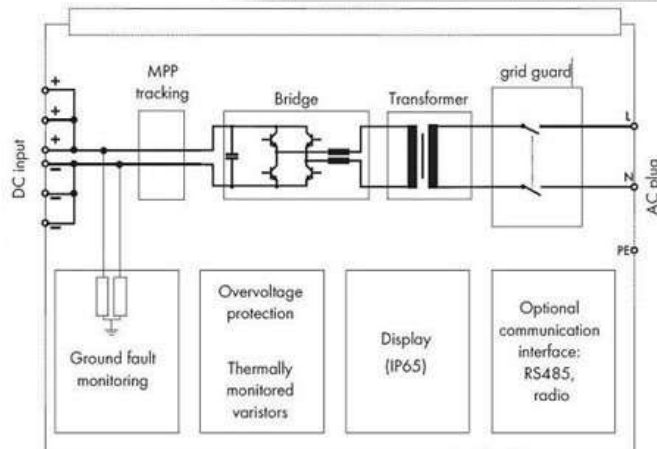
Fig. 12. Schema bloc a unui invertor monofazat cu transformator
