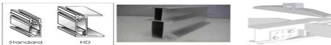
Fig. 22. Sistem fix de montare a panourilor fotovoltaice
