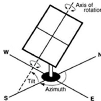
Fig. 29. Schema de principiu a sistemului de orientare pe o axa
