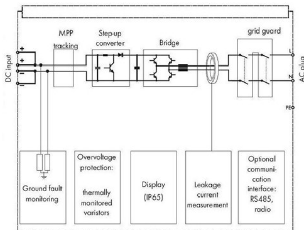
Fig. 11 - Schema bloc a unui inverter monofazat fără transformator
