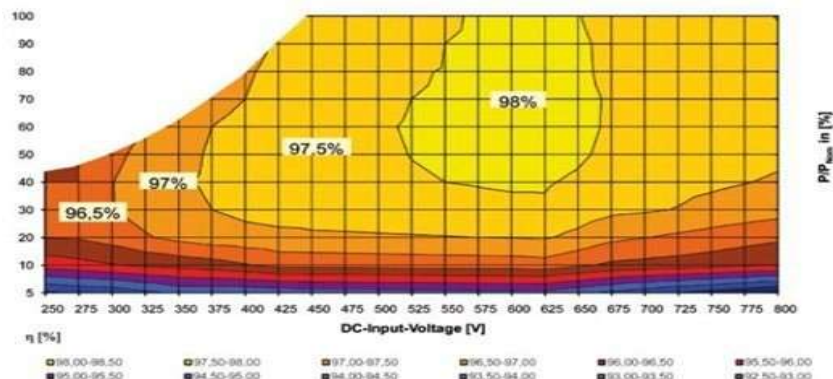
Fig. 14. Randamentul inverterului
