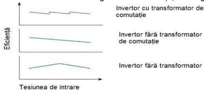
Fig. 13. Eficacitatea diferitelor tipuri de invertore
