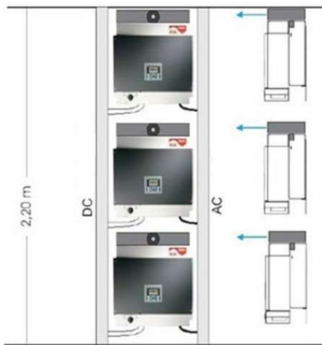
Fig. 16. Invertor cu răcire forțată
