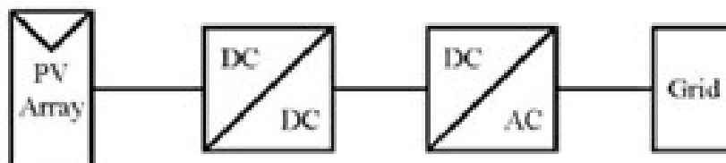
Fig. 10. Schema - bloc a unui invertor fotovoltaic cu convertor ridicător și fără trafa de izolare
