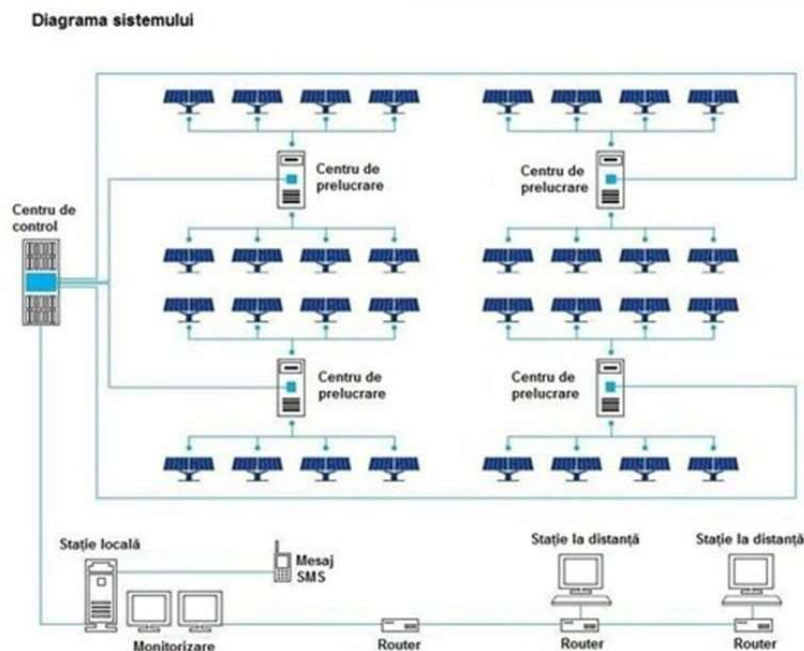
Fig. 34. Monitorizarea centralei fotovoltaice
