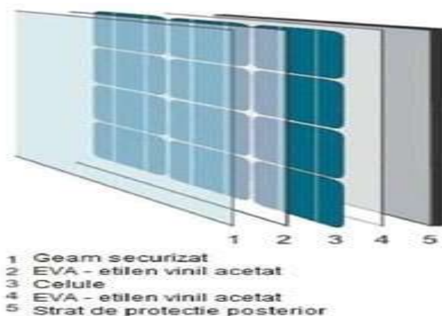
Fig. 6. Structura unui panou solar
